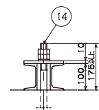
B 矢視図
