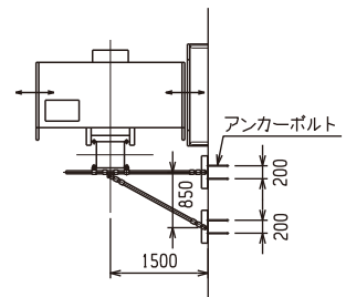
壁つなぎ方法(2)
