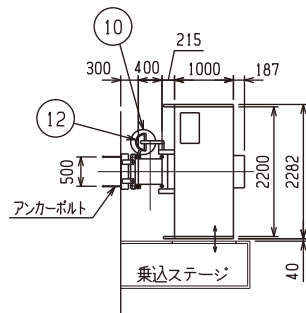
壁つなぎ方法(1)
